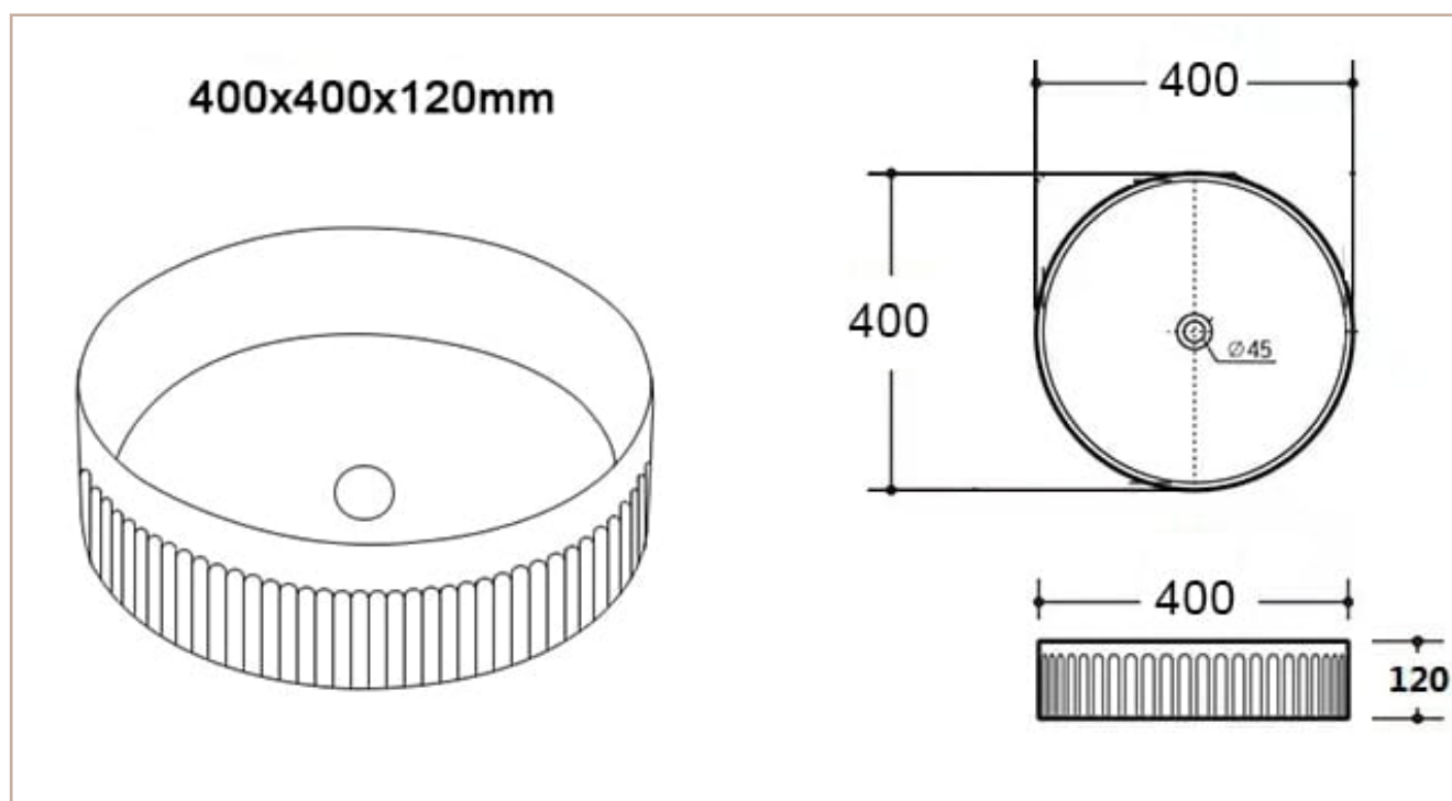
Plan Vasque
