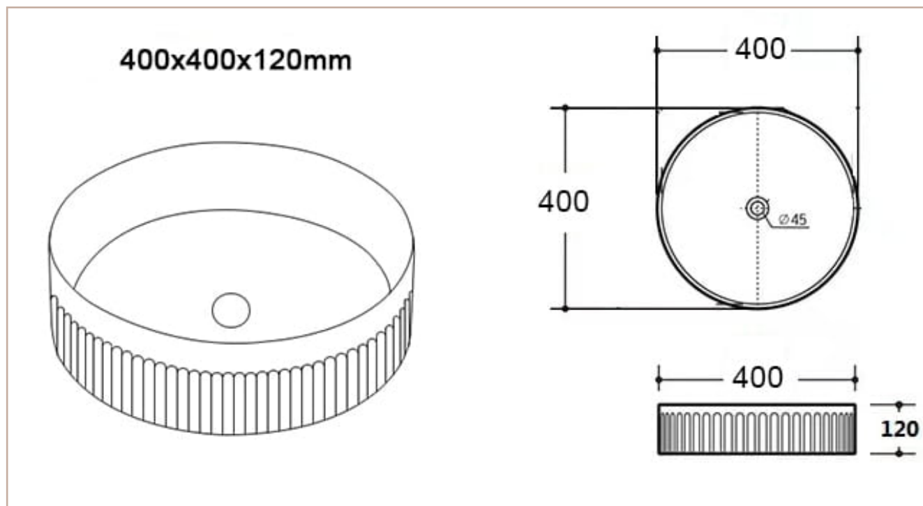
Plan Vasque
