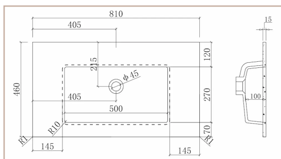
Plan Vasque
