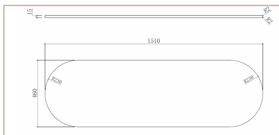
Plan Vasque
