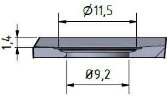
Detalle B
