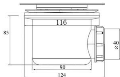
Kit d'évacuation pour série FJORD
