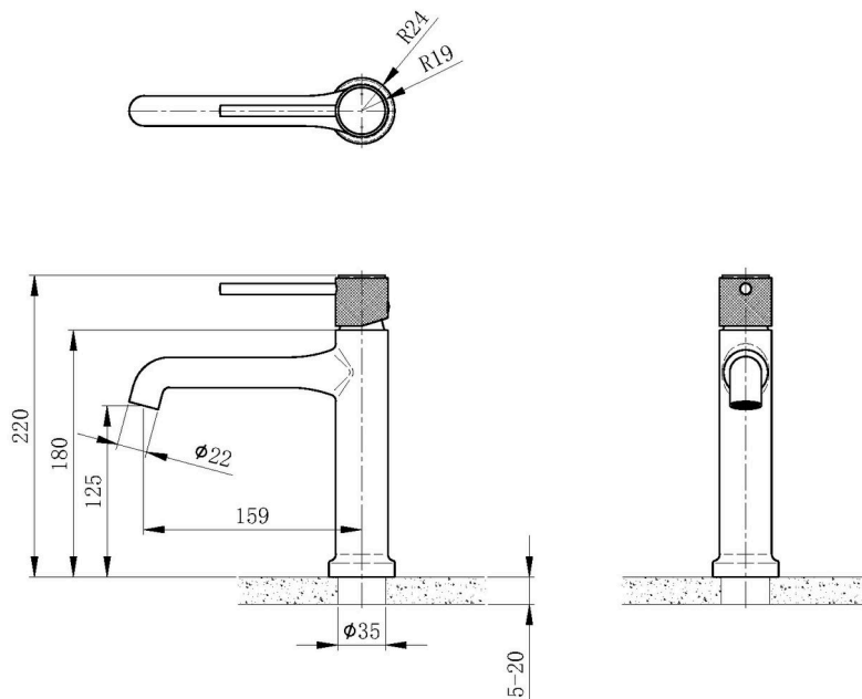
Vue de dessus, de profil et de face · cotes en mm
