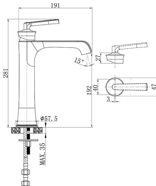
Vue de profil, manette et embase - cotes en mm
