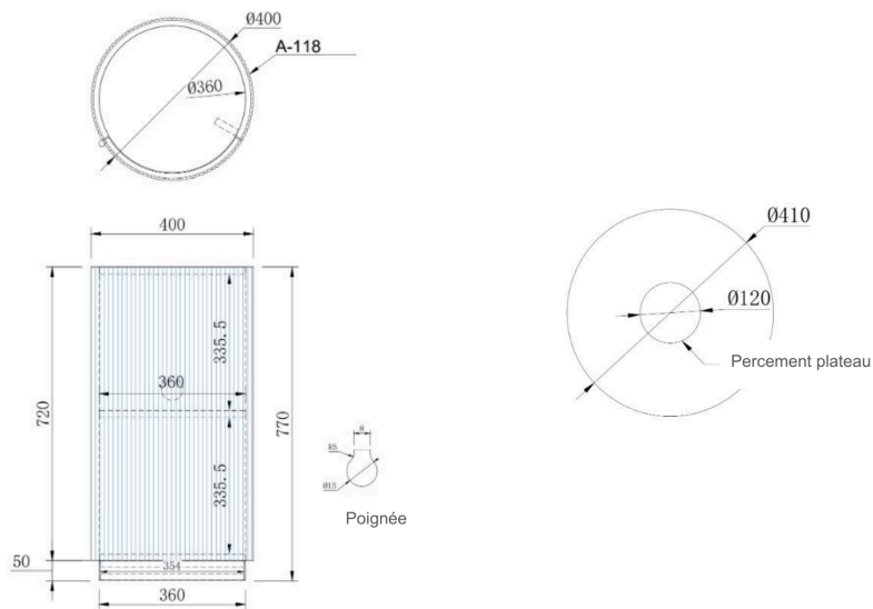
Meuble (dessus et face) et plateau — dimensions en millimètres
