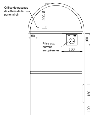
Schéma de structure de face avant
