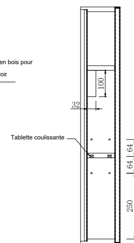
Vue en coupe latérale
