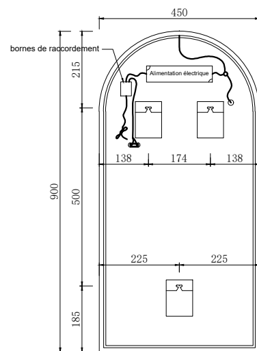
Vue arrière
