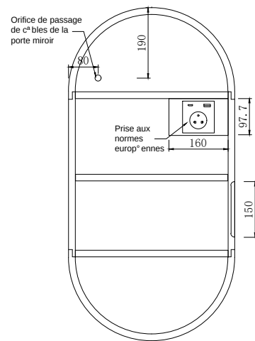
Schéma de structure de face avant
