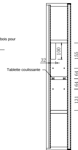
Vue en coupe latérale
